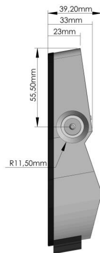
Montaje ESTÁNDAR
